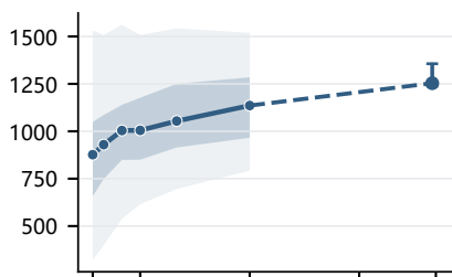
尺度参数 \eta (千次循环)
